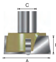
Hinge Boring Bits 開孔取空刀
