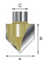
V Groove Bits V型線刀
